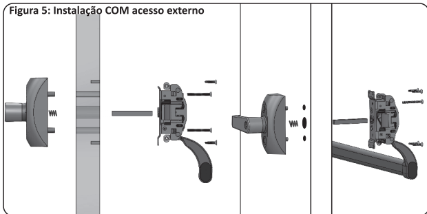
Figura 5: Instalação COM acesso externo
